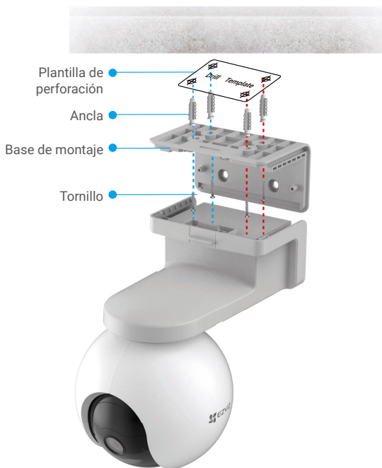
Fig. 1 Montaje en techo
