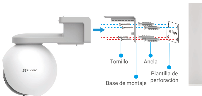
Fig. 2 Montaje en pared
